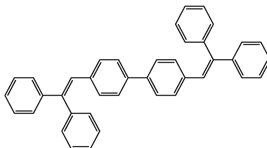
(DPVBi)
