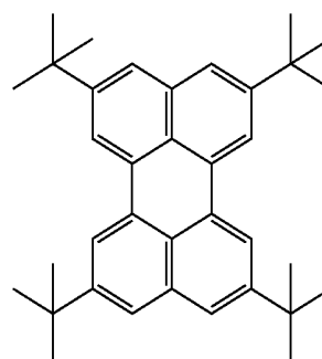
(Tetra-tert-butyl perylene)
